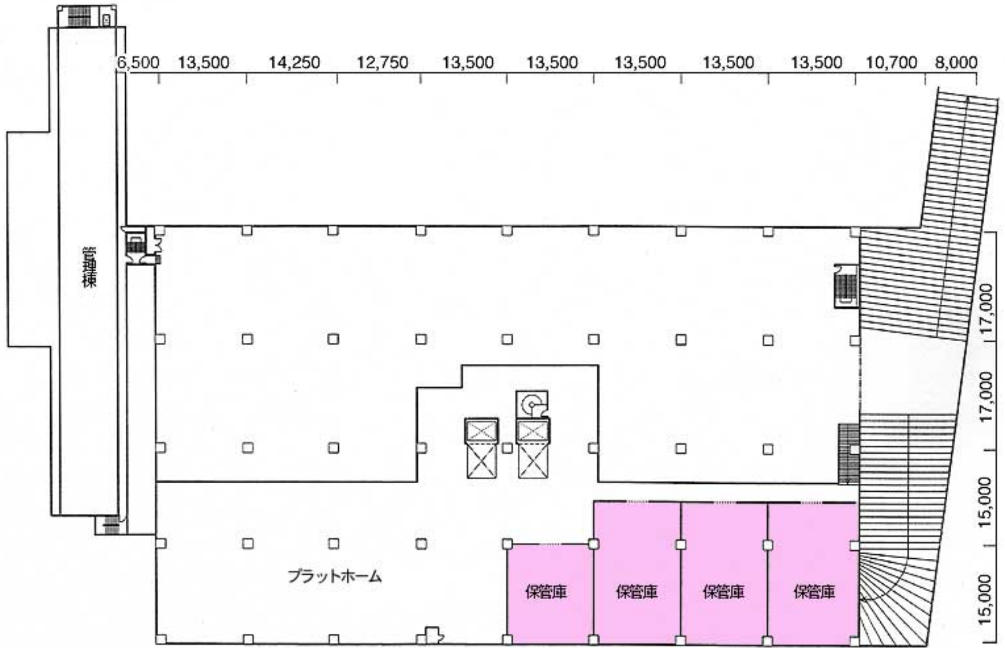
2F平面図
