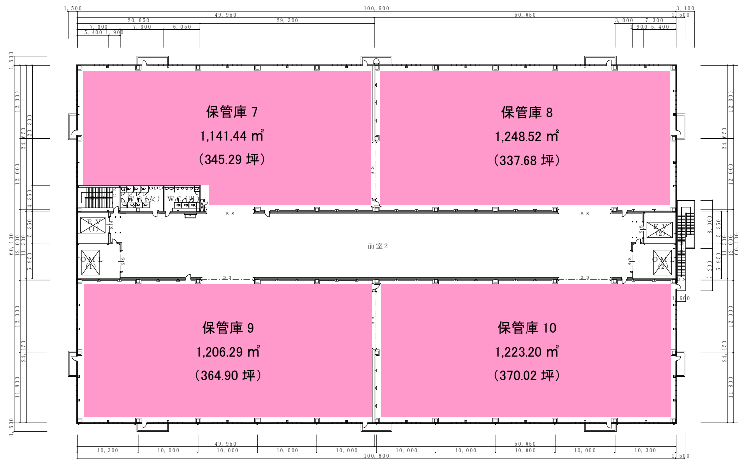
3 階平面図 1 / 200
